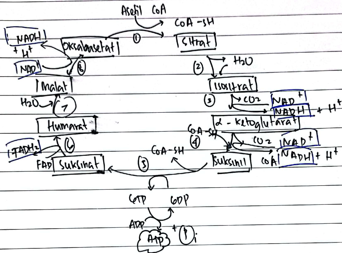
Gambar 2. Siklus krebs.
