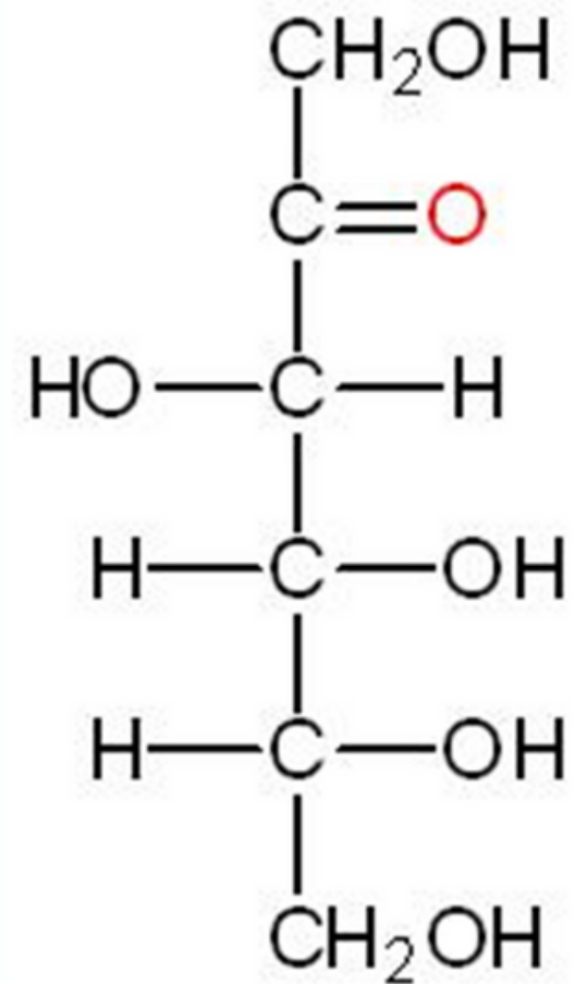
D-fructose
