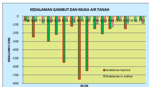
Gambar 5. Kedalaman gambut dan muka air tanah pada beberapa Blok di wilayah kebun Sawit PT. Jalin Vaneo, Kabupaten Kayong Utara
