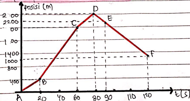
Gratik posisi terhadap waktu
