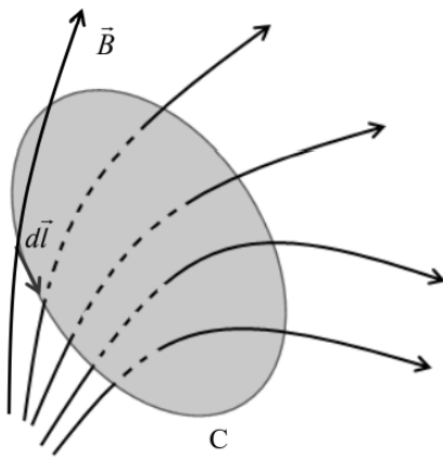
Gambar 5.35 Lintasan tertutup sembarang yang kita simbolkan dengan C dalam ruang yang mengandung medan magnet.
