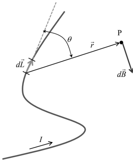
Gambar 5.1 Elemen kawat yang dialiri arus listrik menghasilkan medan magnet di sekitarnya. Medan magnet total di suatu titik samam dengan jumlah medan magnet yang dihasilkan oleh semua elemen tersebut. Karena medan magnet adalah besaran vector maka penjumlahan dilakukan secara vector.
