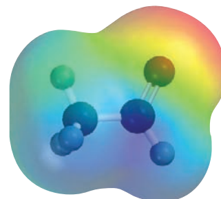
CH 3 CHO
