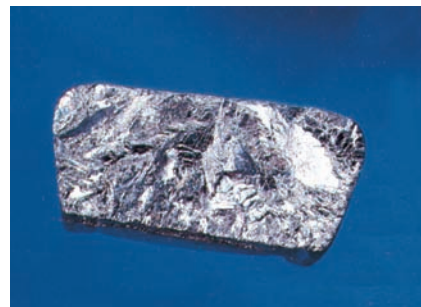
Bismuth (Bi)
