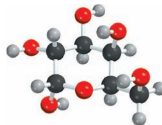
C 6 H 12 O 6
